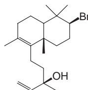
3-Bromo-7,14-labdadiene-13-ol
