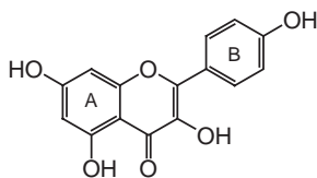
Kaempferol
