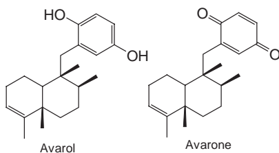
Avarol
